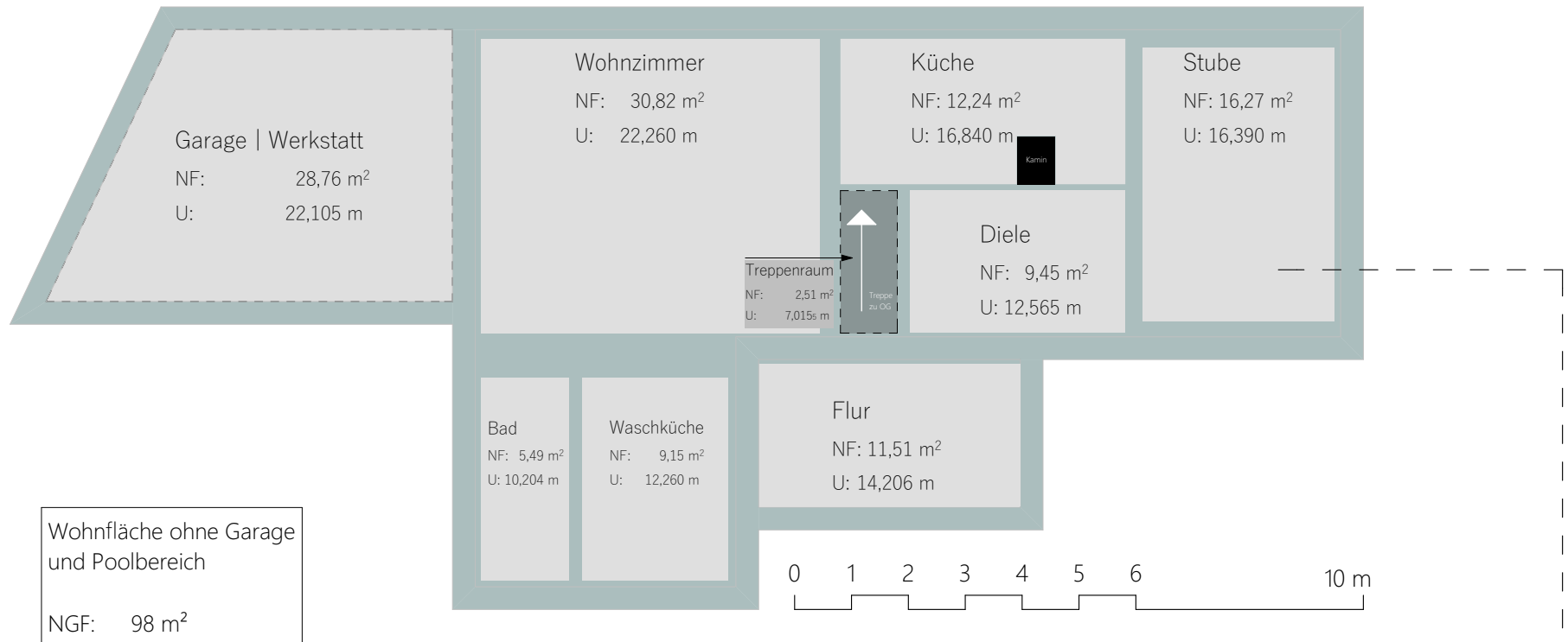
Wohnfläche Erdgeschoss
